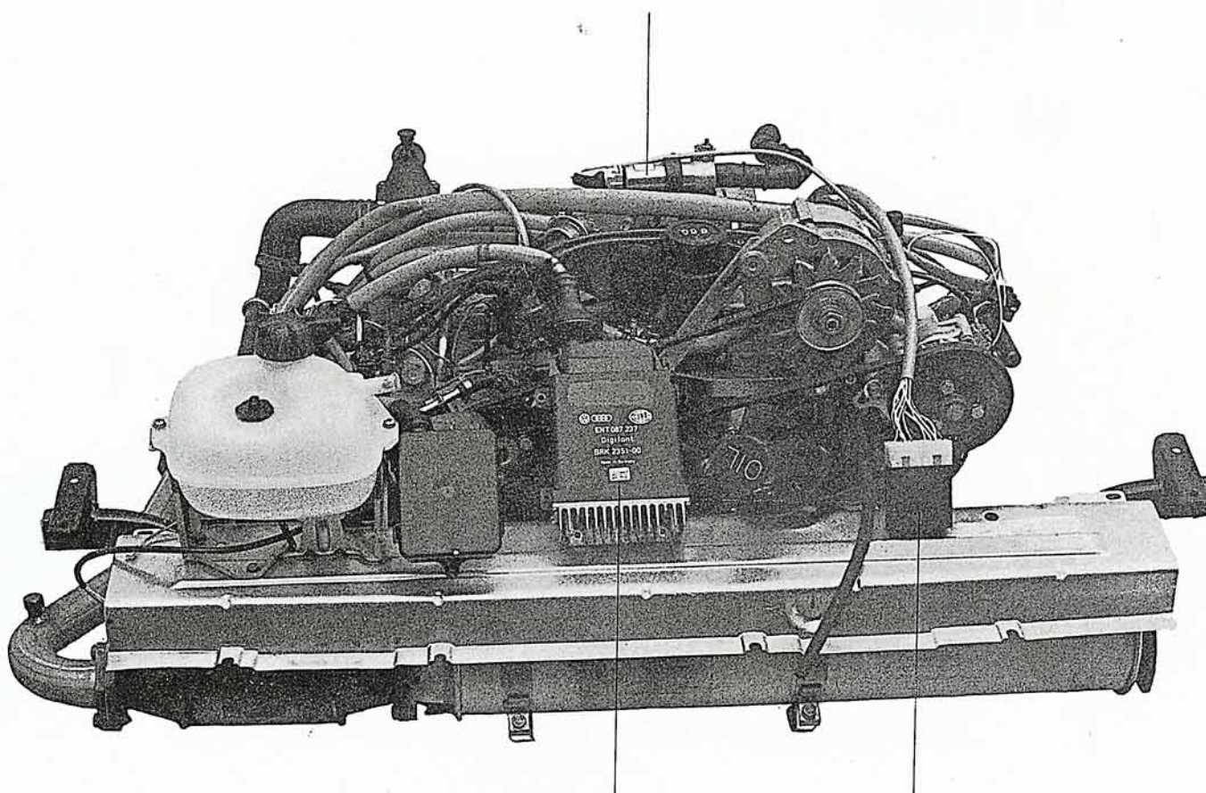
Steuergerät/Digifant
