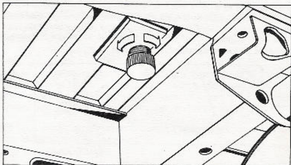
Robinet de vidange du réservoir d'eau
