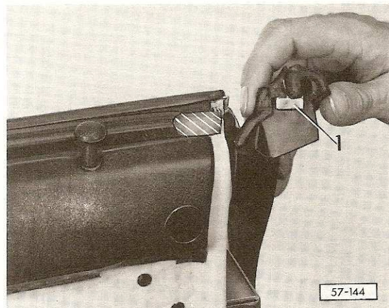
Fig. 3 Joint de porte: dépose
