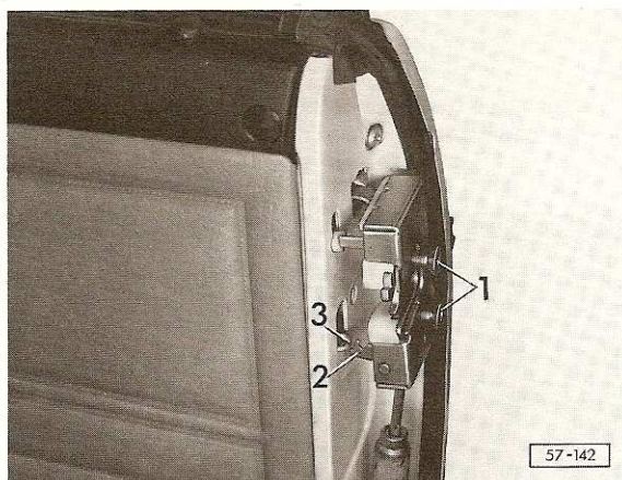
Fig. 1 Serrure de porte: dépose
