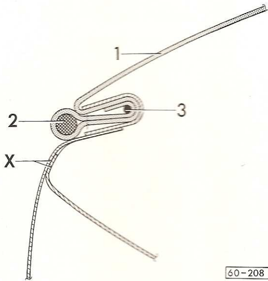
Schéma: garniture de capote sur la carrosserie
