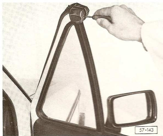
Fig. 2 Joint de porte: dépose
