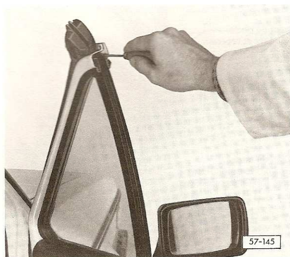
Fig. 4 Rail de guidage: dépose
