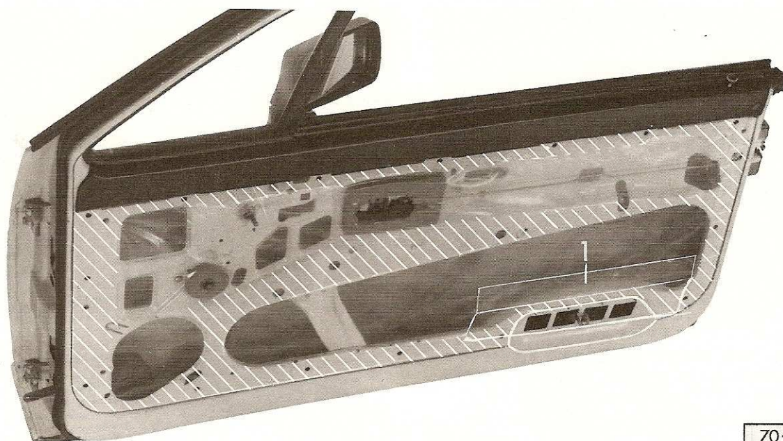
Fig. 1 Feuille de protection de revêtement de porte: remplacement
